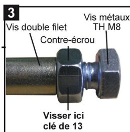
Mettre la vis TH + l'écrou sur la vis double filet pour faire contre-écrou.
