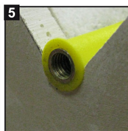
Débloquer l'écrou, dévisser le fond du contre-écrou. La cheville est prête à recevoir la pièce à fixer.
