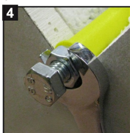
Visser la vis double filet à fond (clé plate de 13). Voir photo n°5
