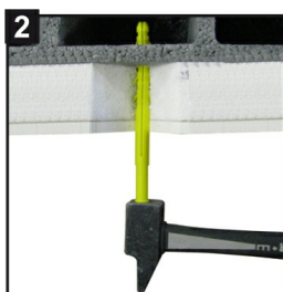
Enfoncer la cheville entièrement au ras de la plaque de plâtre à l'aide d'un marteau.
