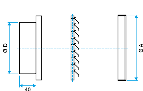
Grille AR 637 diamètre 125 à 315 mm
