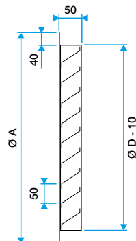
Grille AR 637 diamètre 400 à 630 mm
