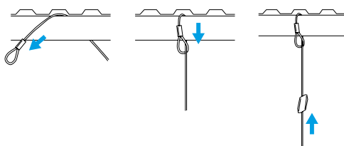
Schéma d'installation des câbles de suspension rapide
