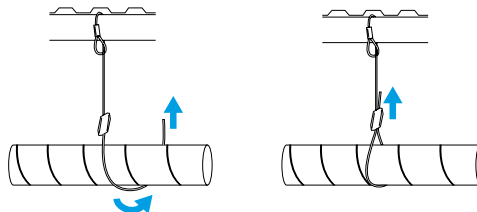
Schéma d'installation des câbles de suspension rapide
