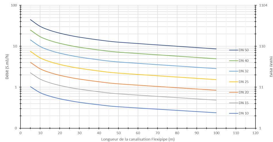
Capacité de débit Gaz Naturel H 21 mbar - \Delta P 1 mbar
