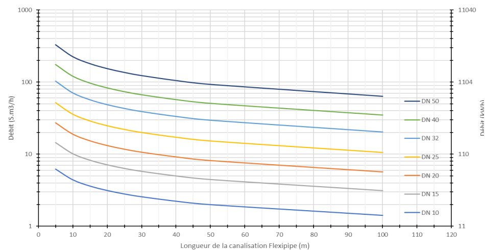
Capacité de débit Gaz Naturel H 300 mbar - \Delta P 10%
