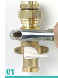
01 Monter le raccord FLEXICLIC sur le robinet
