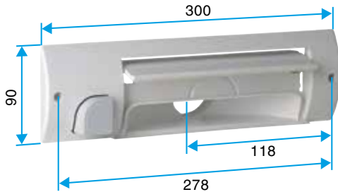
Encombrement plinthe ramasse-miettes
