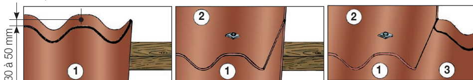
Complément d'étanchéité longitudinal
