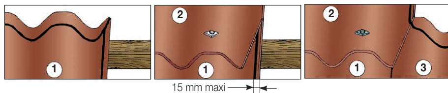
Complément d'étanchéité longitudinal
